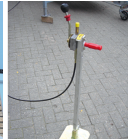
Bowdenzugfernbedienung
